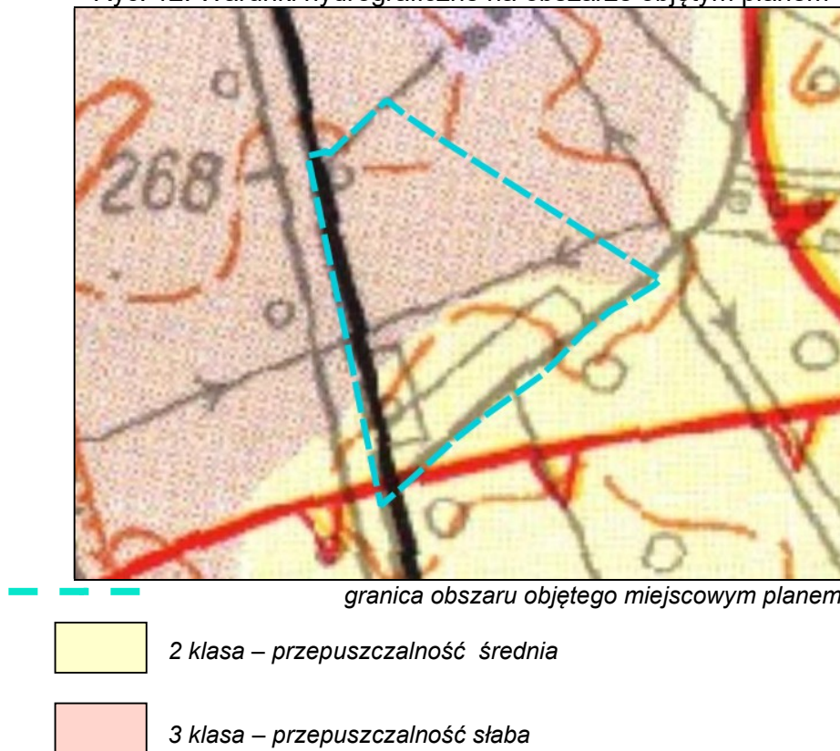
Ryc. 12. Warunki hydrograficzne na obszarze objętym planem
